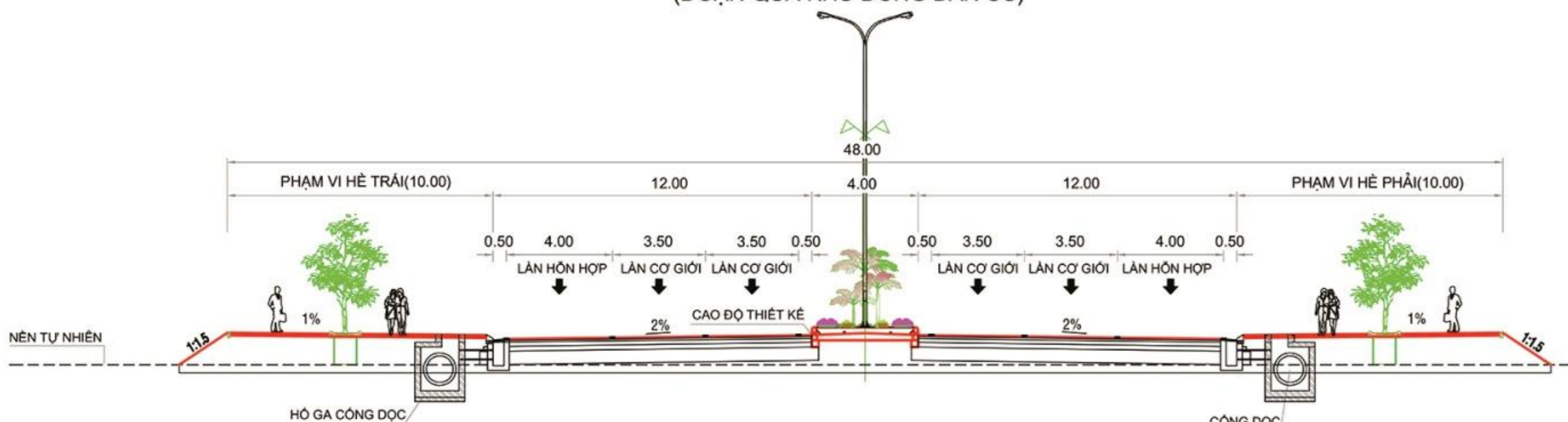
MẶT CẮT NGANG ĐIỂN HÌNH (ĐOẠN QUA KHU ĐÔNG DÂN CƯ)
