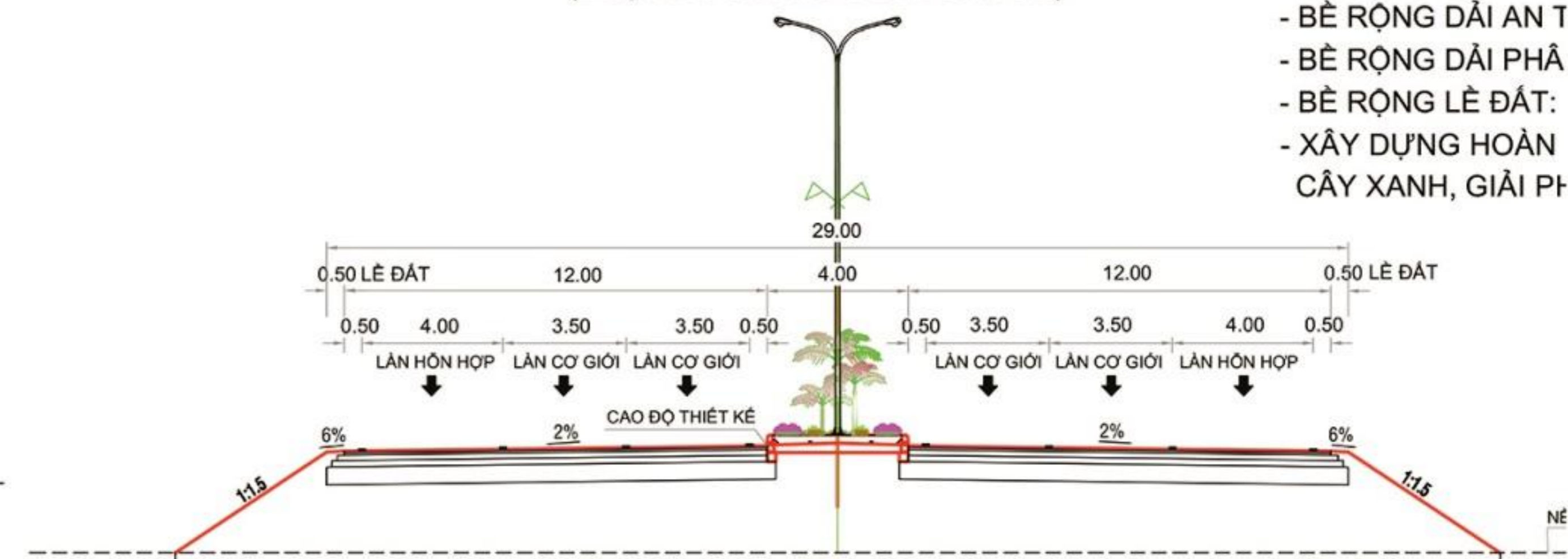
MẶT CẮT NGANG ĐIỂN HÌNH (ĐOẠN NGOÀI KHU ĐÔNG DÂN CƯ)
